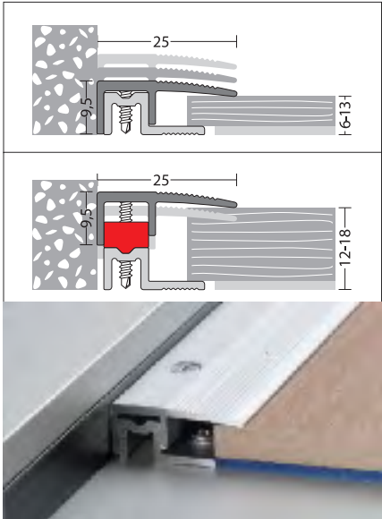
Abschlussprofil PS400PEP Geschraubtes, zweiteiliges Aluminiumprofil, z.B. für Wandabschlüsse. Für Belagstärken von 6 – 13 mm 25 mm × 1 m | 2,7 m Verpackungseinheit: 10 Stück/Karton Mindestbestellmenge: 1 Stück
