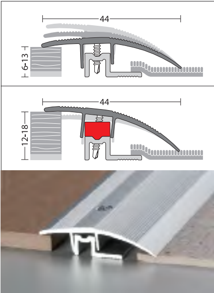
Anpassungsprofil PS400PEP Geschraubtes, zweiteiliges Aluminiumprofil für Übergänge zwischen unterschiedlich hohen Bodenbelägen. Für Belagstärken von 6 – 13 mm 44 mm × 1 m | 2,7 m Verpackungseinheit: 10 Stück/Karton Mindestbestellmenge: 1 Stück
