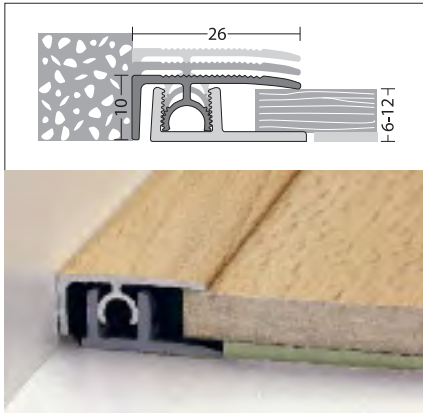
Abschlussprofil Profitec Junior Zweiteiliges Aluminiumprofil, z.B. für Wandabschlüsse. Für Belagstärken von 6 – 12 mm 26 mm × 1 m | 2,7 m Verpackungseinheit: 10 Stück/Karton Mindestbestellmenge: 1 Stück
