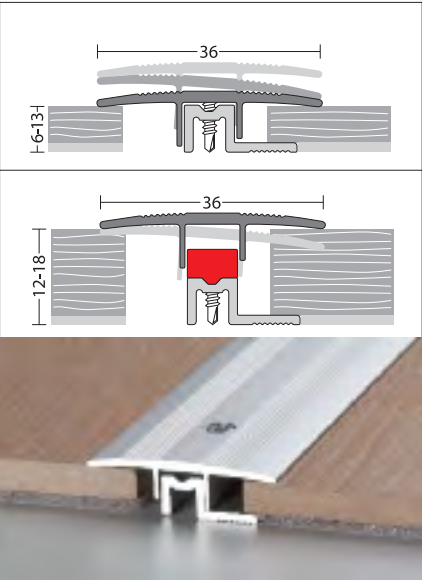
Übergangsprofil PS400PEP Geschraubtes, zweiteiliges Aluminiumprofil zur Überdeckung von Dehnungsfugen. Für Belagstärken von 6 – 13 mm 36 mm × 1 m | 2,7 m Verpackungseinheit: 10 Stück/Karton Mindestbestellmenge: 1 Stück
