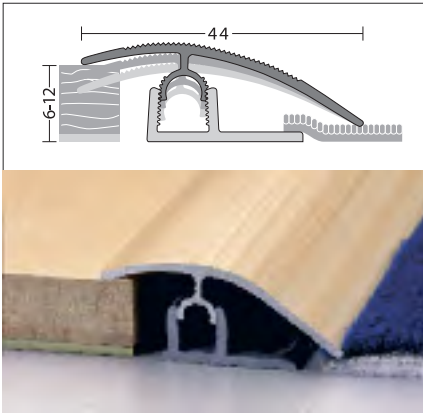
Anpassungsprofil Profitec Junior Zweiteiliges Aluminiumprofil für Übergänge zwischen unterschiedlich hohen Bodenbelägen. Für Belagstärken von 6 – 12 mm 44 mm × 1 m | 2,7 m Verpackungseinheit: 10 Stück/Karton Mindestbestellmenge: 1 Stück
