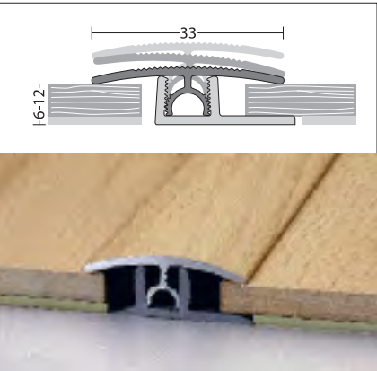
Übergangsprofil Profitec Junior Zweiteiliges Aluminiumprofil zur Überdeckung von Dehnungsfugen. Für Belagstärken von 6 – 12 mm 33 mm × 1 m | 2,7 m Verpackungseinheit: 10 Stück/Karton Mindestbestellmenge: 1 Stück
